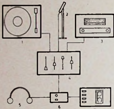
Fig. 8. Combinatie mogelijkheid met de meeluisterversterker.
